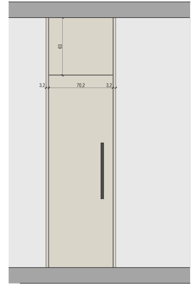
Z6_POZ 01.1 C-C 1:20
