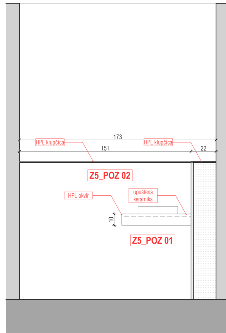
ZONA 5 B-B 1:20
