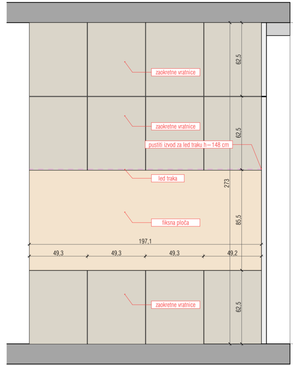
Z6_POZ 01 A-A 1:20
