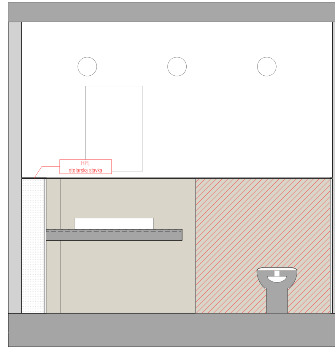
ZONA 5 A-A 1:20
