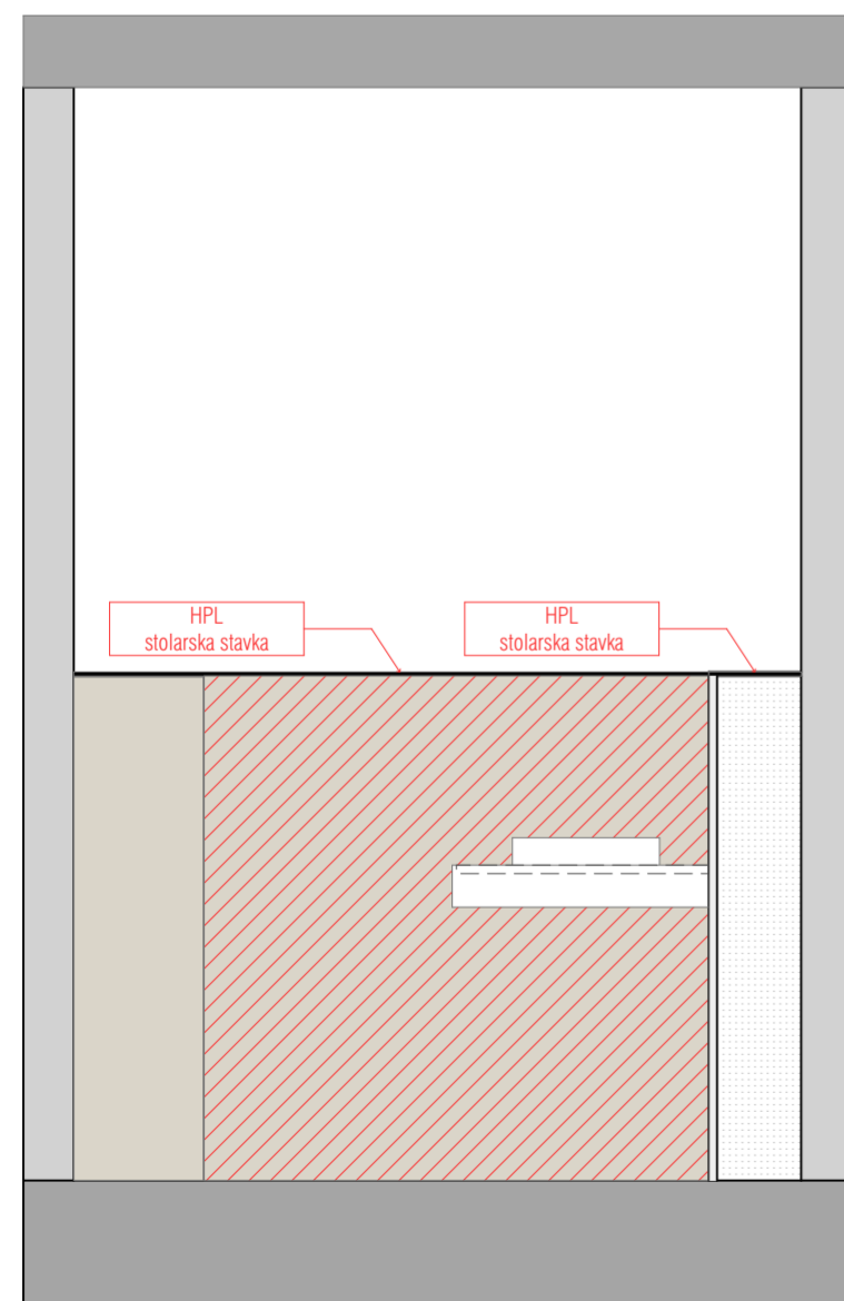
ZONA 5 B-B 1:20
