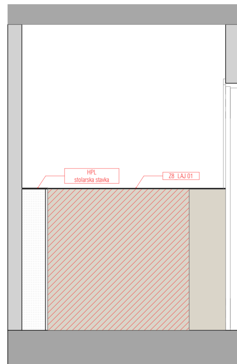
ZONA 5 C-C 1:20
