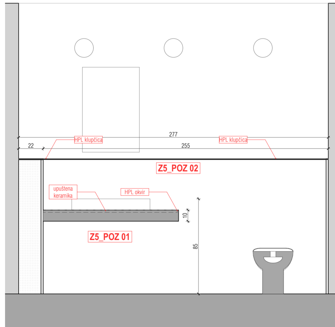
ZONA 5 A-A 1:20
