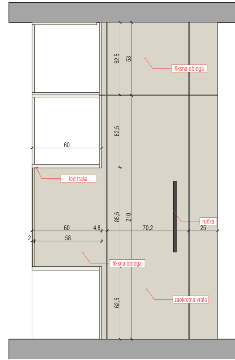
Z6_POZ 01 / Z6_POZ 01.1 B-B 1:20
