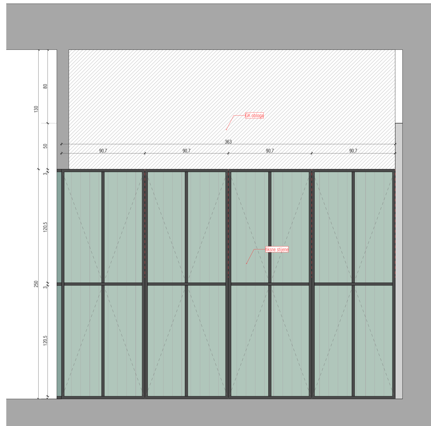
Z3_BR 03
