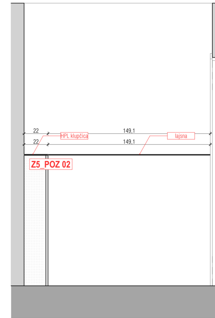
ZONA 5 C-C 1:20
