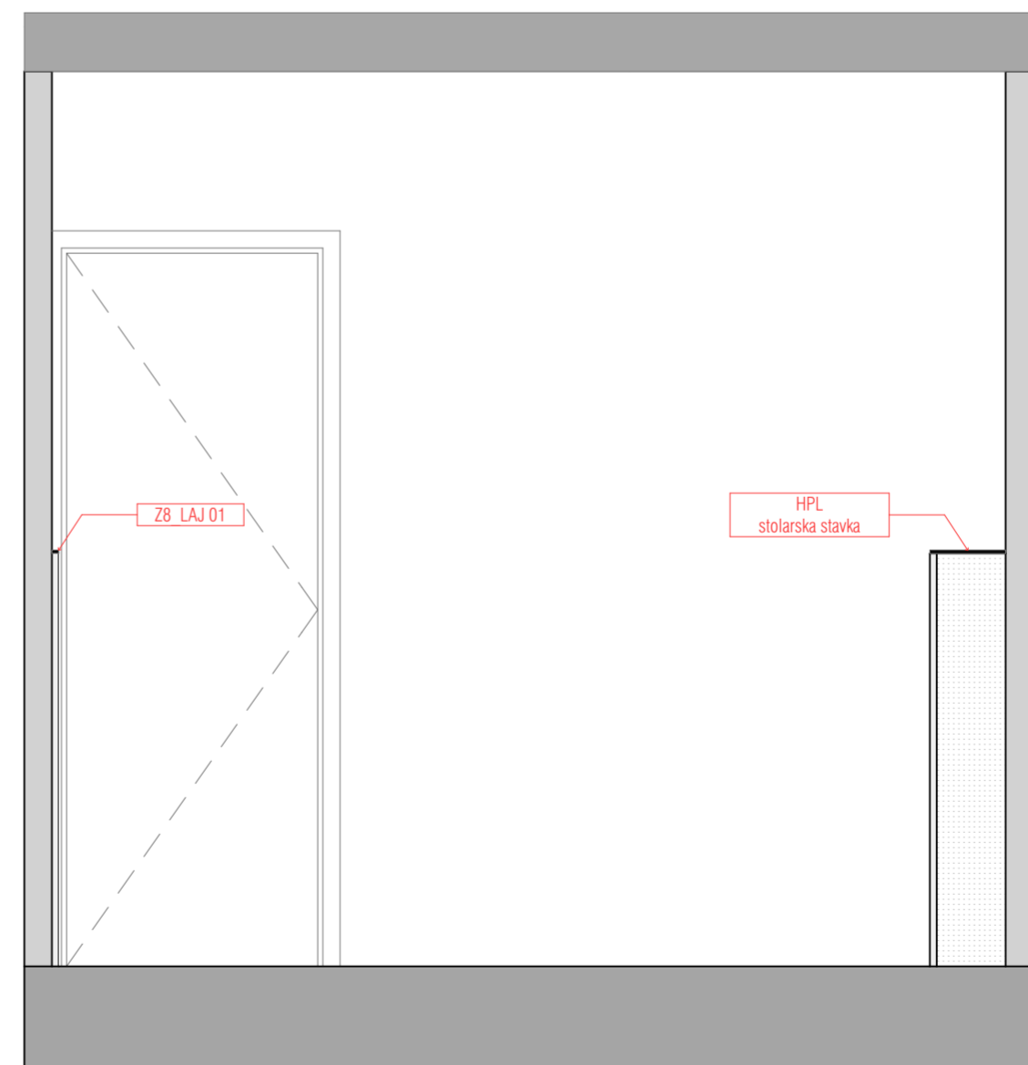
ZONA 5 D-D 1:20
