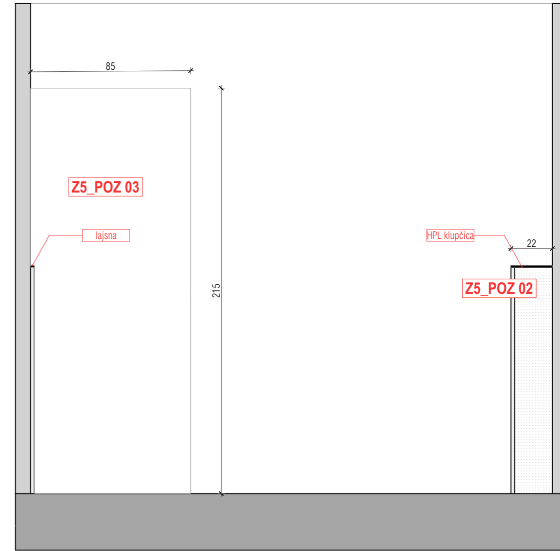
ZONA 5 D-D 1:20
